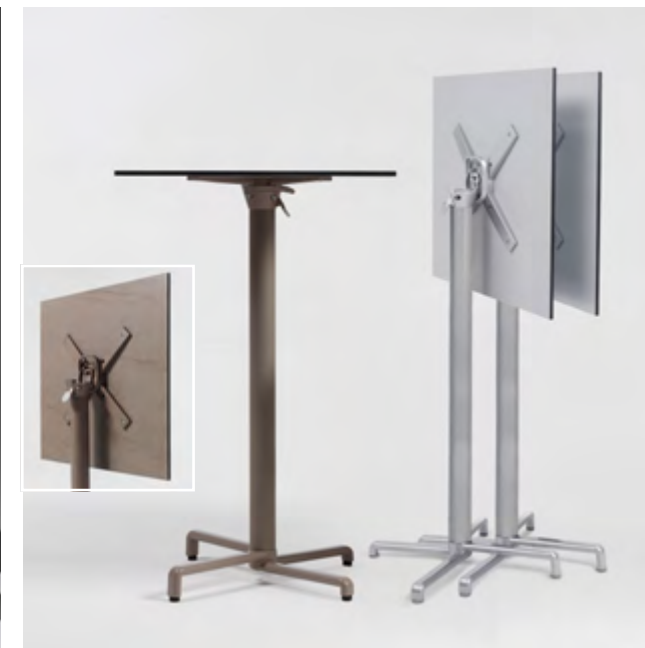
BR93 Basamento bar pieghevole ed accatastabile, ideale per esterno-interno in alluminio verniciato nei colori a scelta, colonna tonda, base dotata di piedini regolabili. Possibilità a richiesta di trattamento speciale per ambienti ad alto tasso salino, disponibile in 2 altezze.
