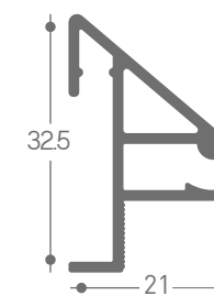
Profilo di alluminio Aluminium profile
